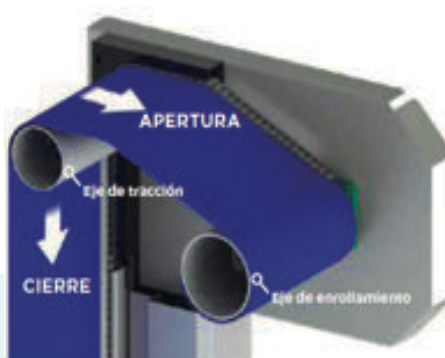
Sistema de transmisión y enrollamiento B-DRIVE CP
