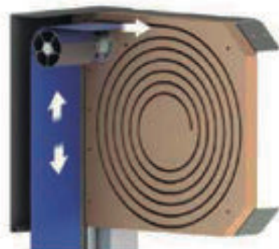
Sistema de transmisión y enrollamiento B-DRIVE SP
